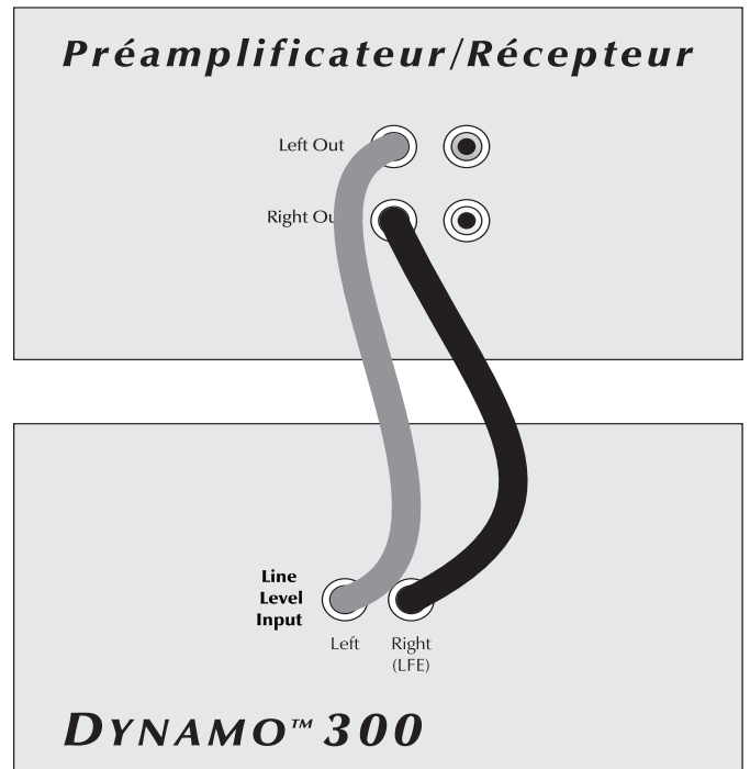
Figure 3. Raccord de signal pour le mode à deux canaux par l'entrée de niveau de ligne.
